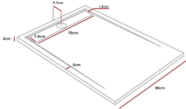
BONDE 90° HORIZONTALE / HORIZONTAL DRAIN 90°
