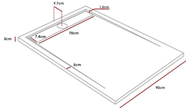
BONDE 90° HORIZONTALE / HORIZONTAL DRAIN 90°
